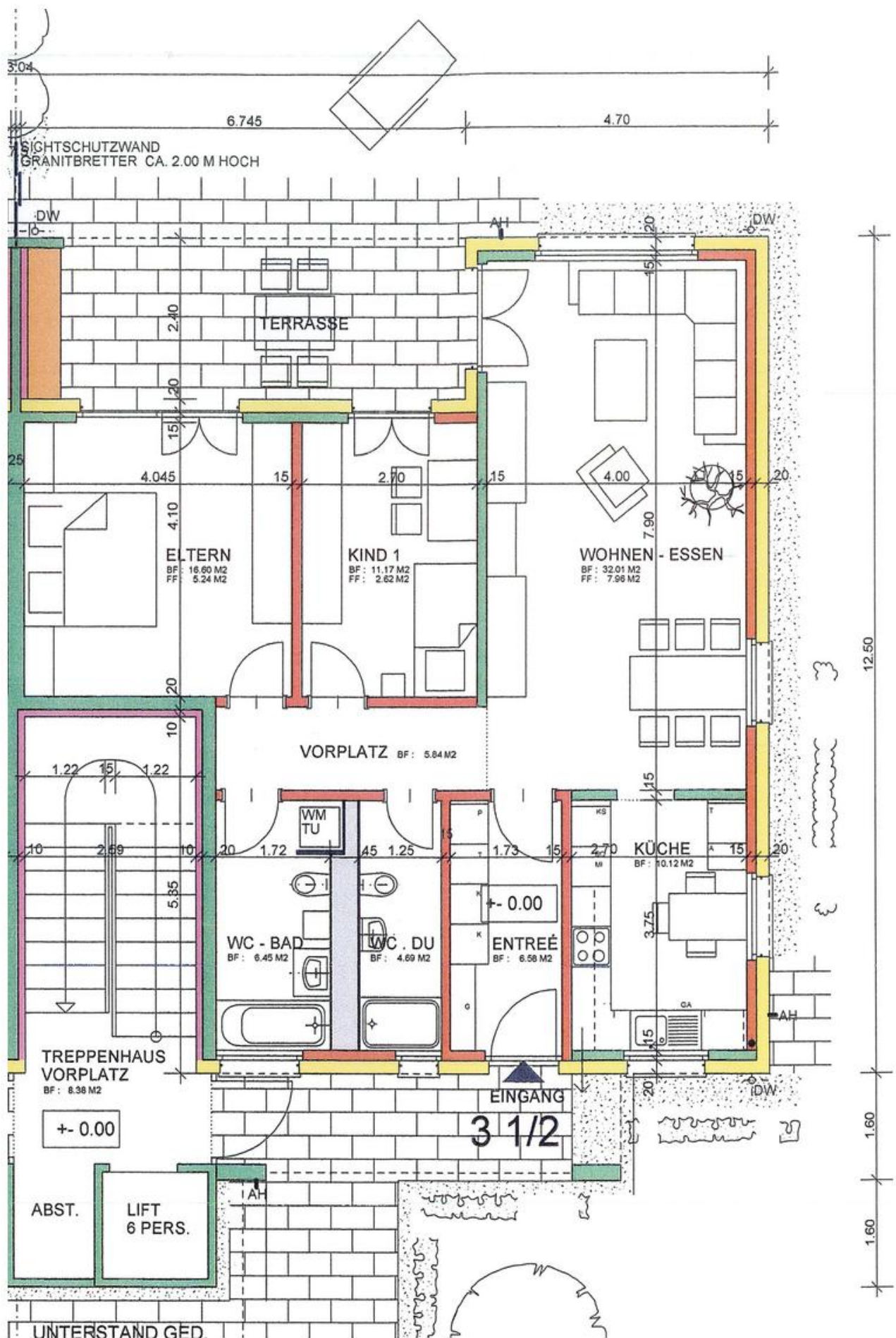
Grundriss 3.5 Zi. Wohnung, EG
