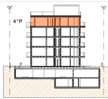
SEZIONE
