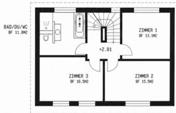
OBERGESCHOSS
