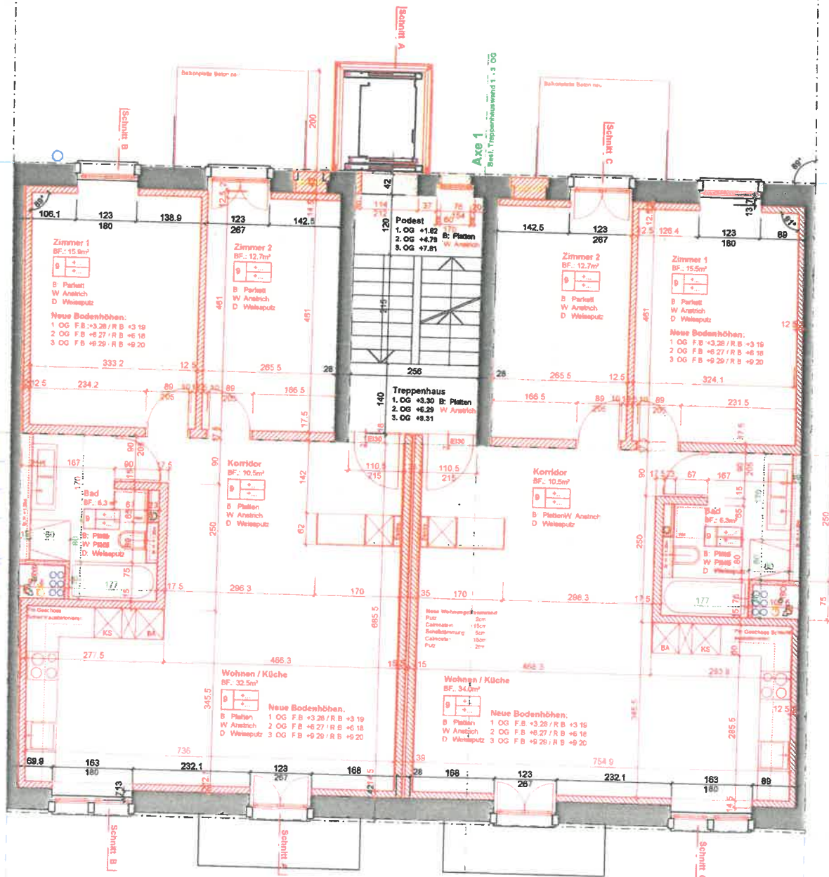
1.-3. Obergeschoss Werkplan
