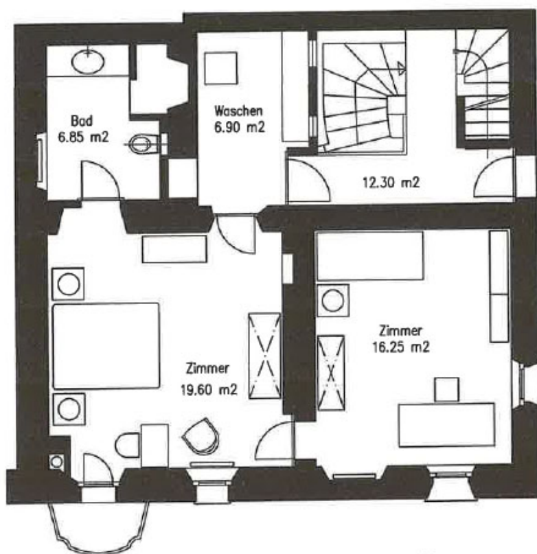
1. Obergeschoss Mst. 1:100
