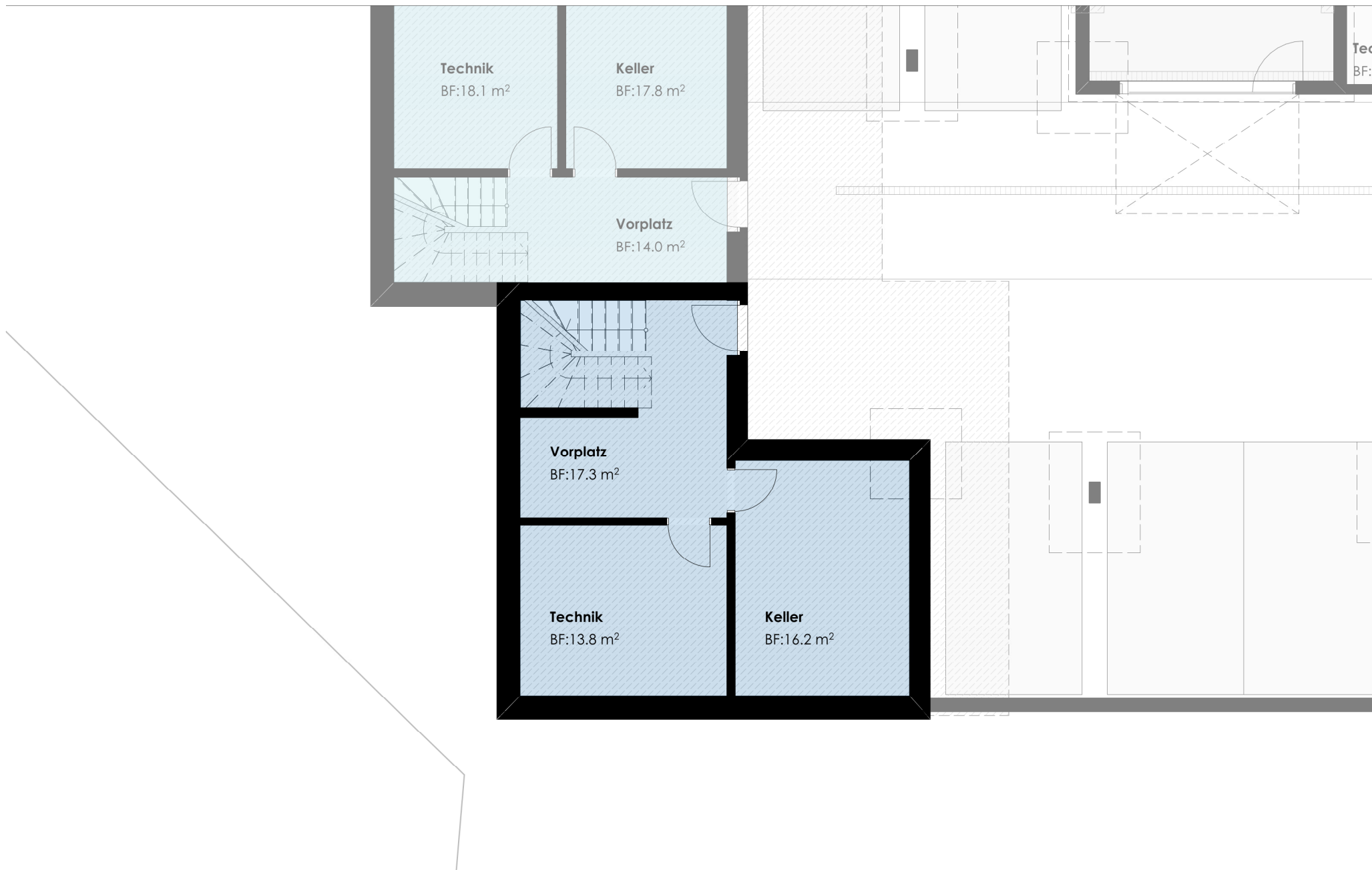
Haus C2 Grundriss Untergeschoss
