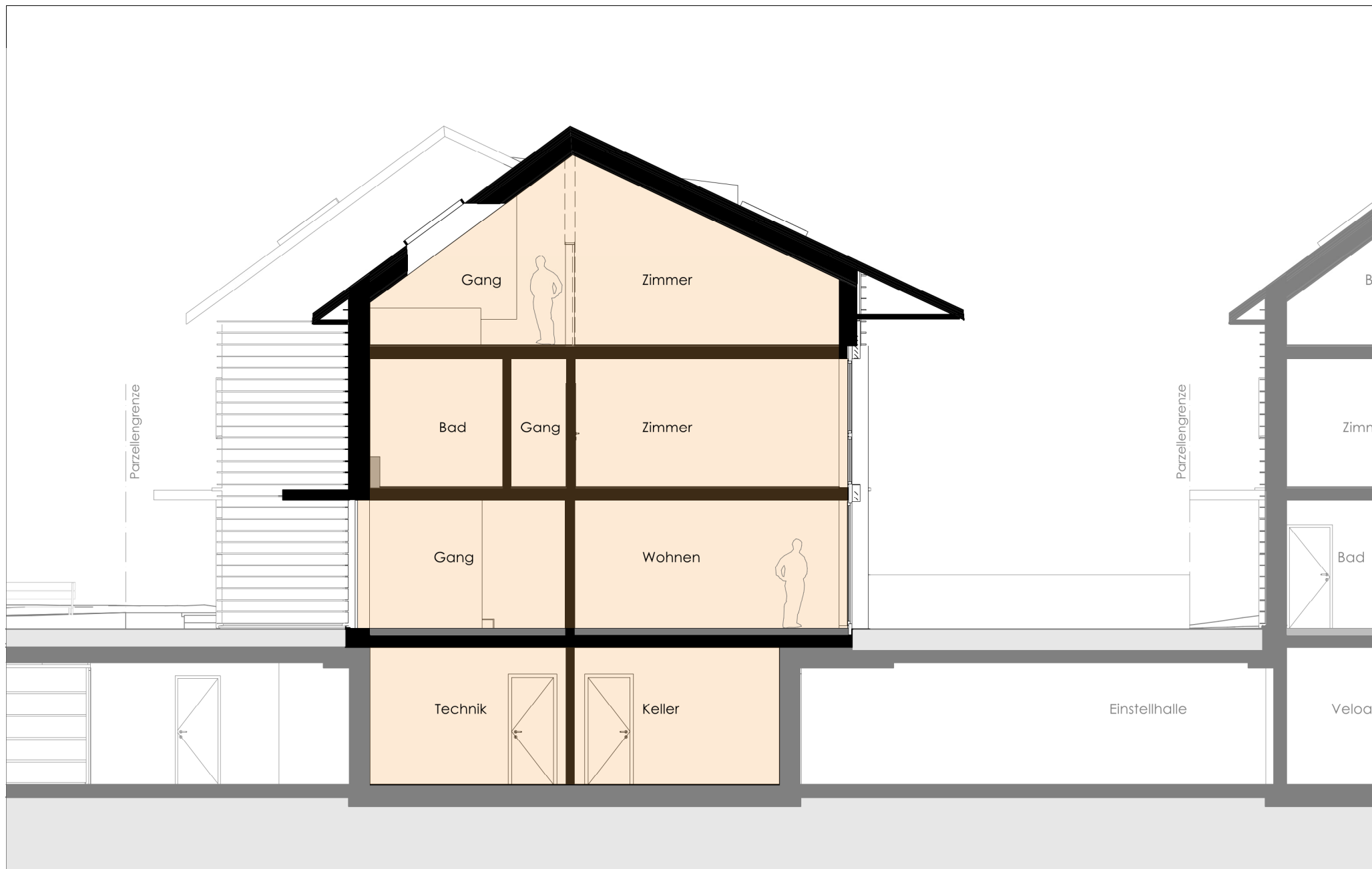
Haus B2 Querschnitt
