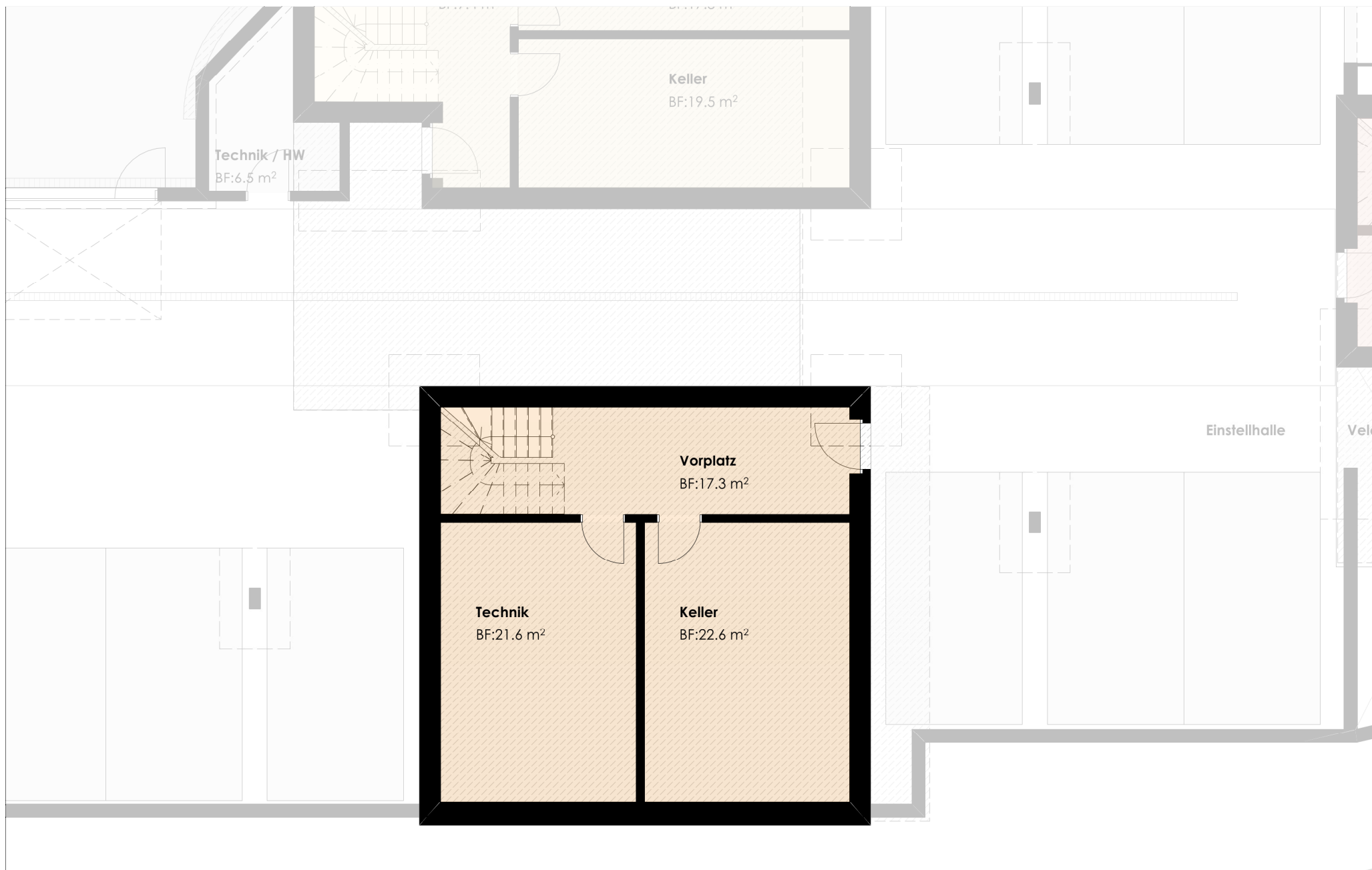
Haus B2 Grundriss Untergeschoss
