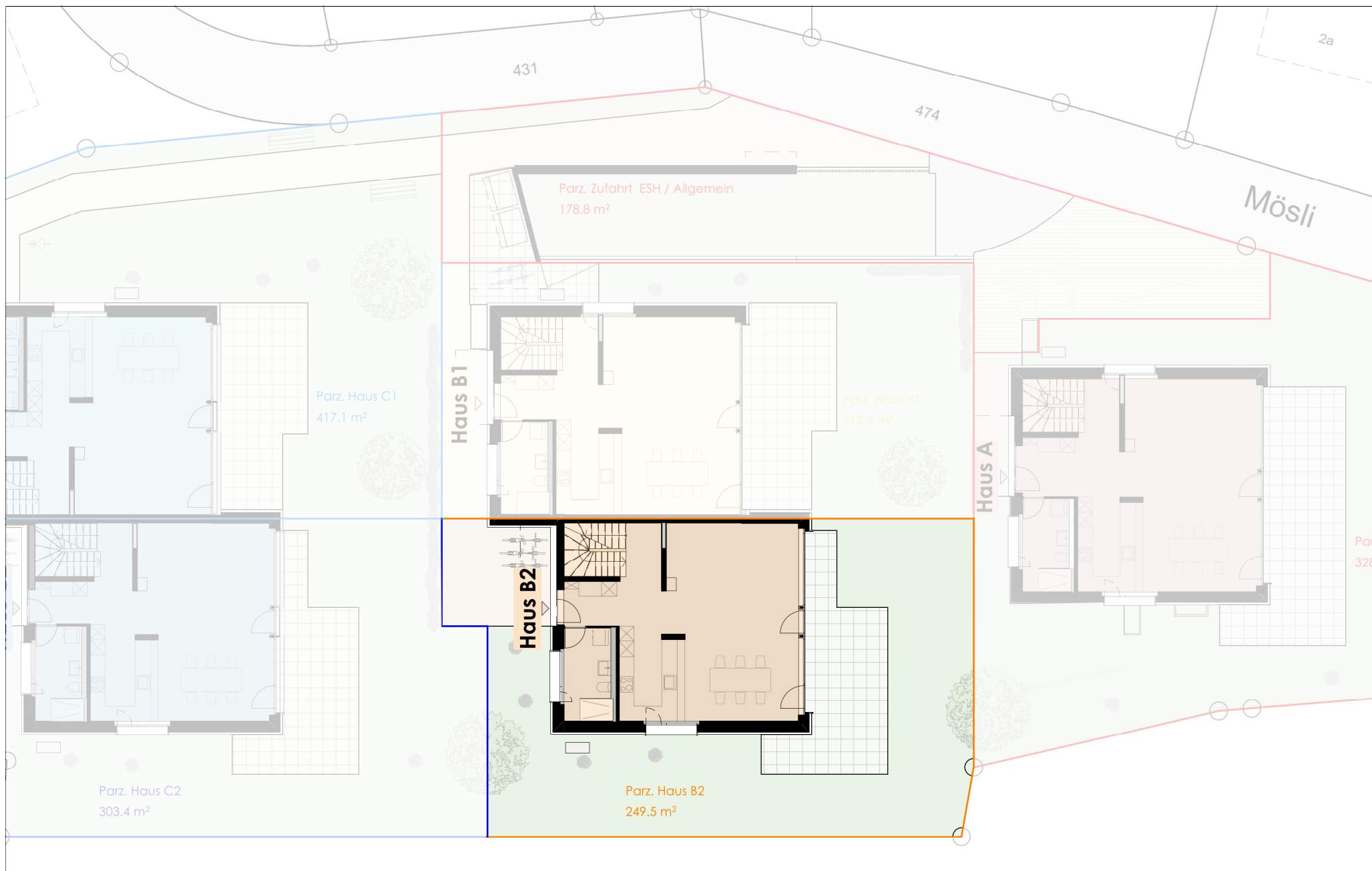
Haus B2 Grundriss EG mit Umgebung
