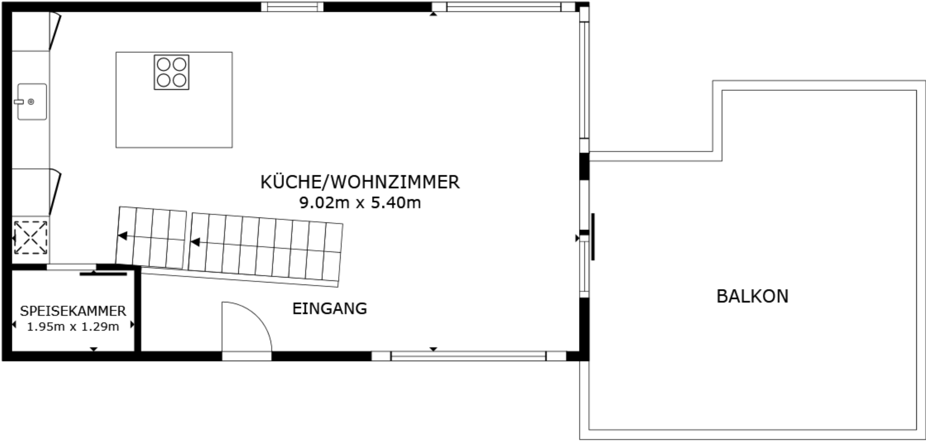
STOCKWERK 2
