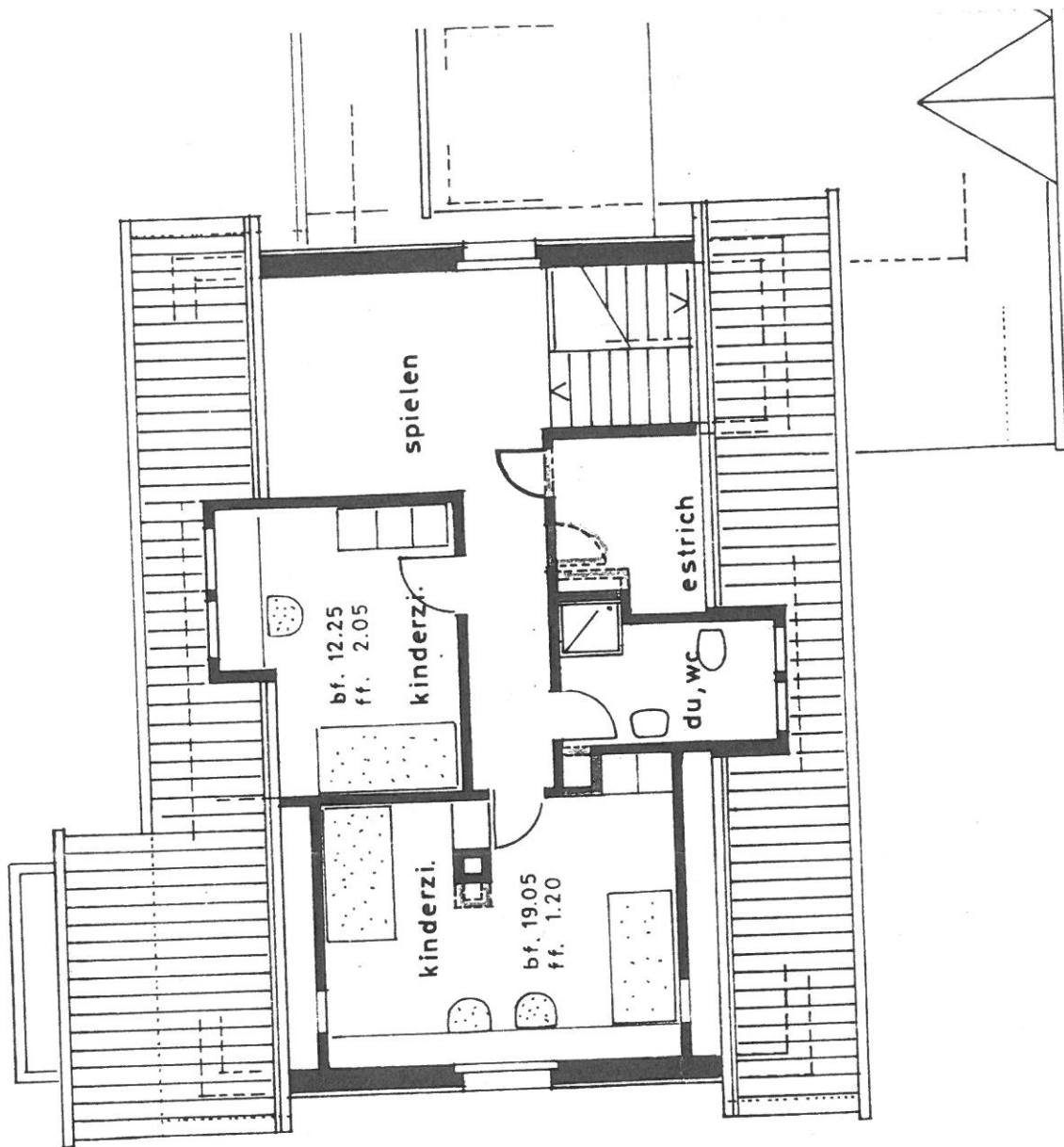
dachgeschoss
